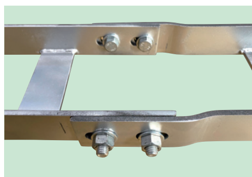
標準仕様の鋼製ケーブルラック
